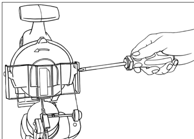
Рис.17 Снятие защиты
